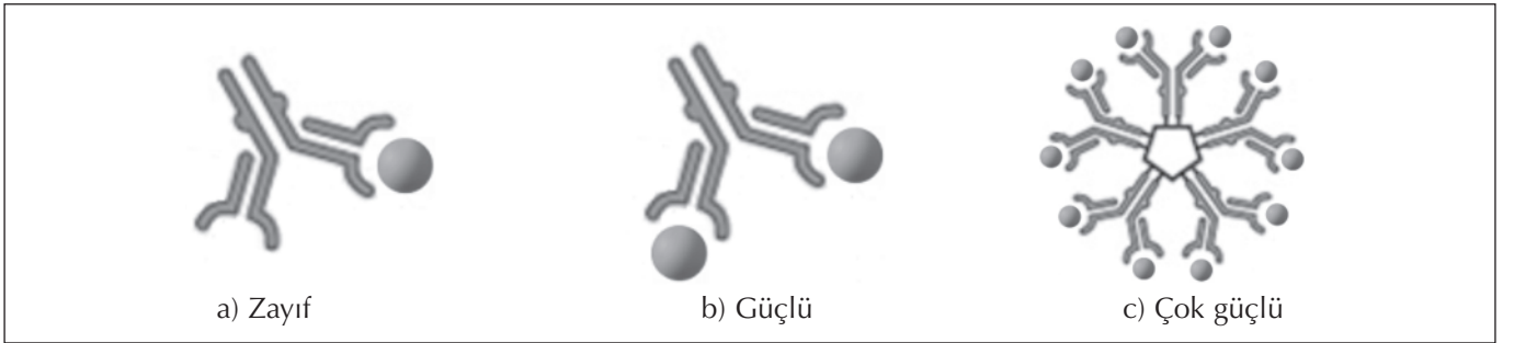
Şekil-5: Afinite-Avidite
